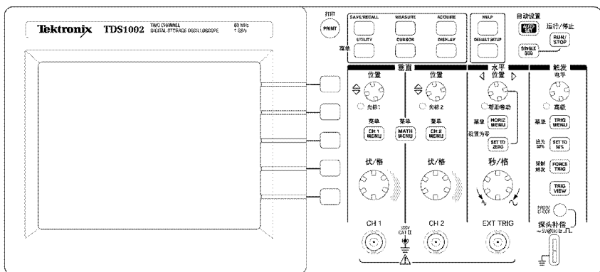
2 通道型
